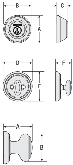
KNOB DIMENSIONS
